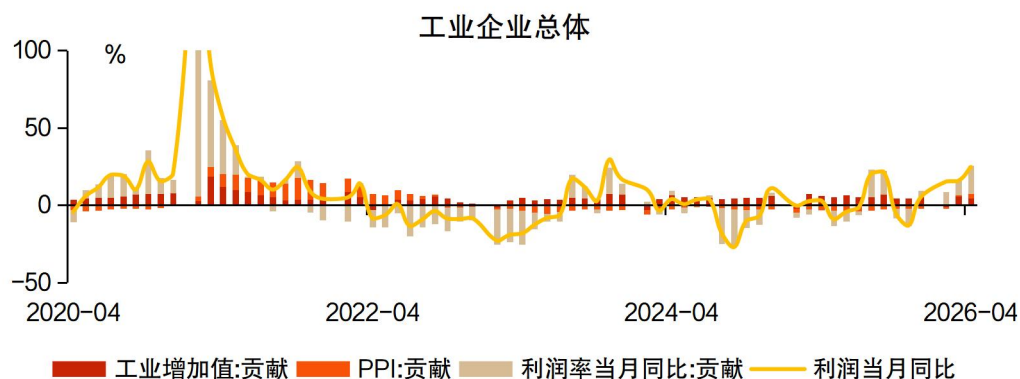
图表 4：利润三因子拆分来看，4 月“利”贡献明显扩大
