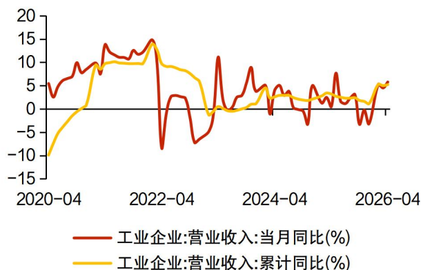
图表 3：4 月营收当月同比小幅改善
