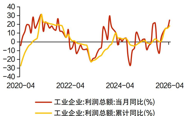
图表 2：4 月利润当月同比延续上行
