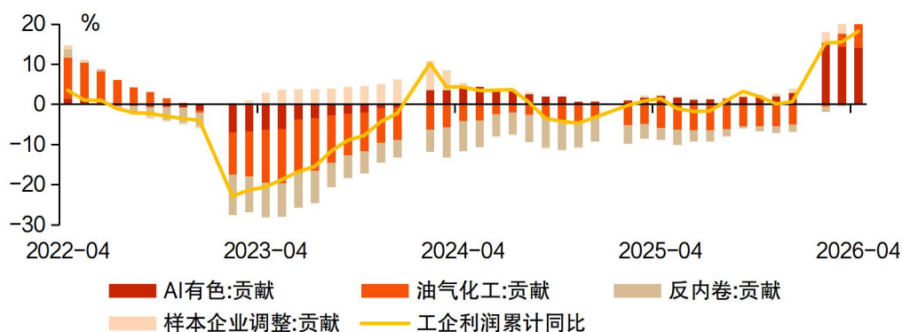
图表 8：分链条来看，4 月油气化工链的贡献明显扩大
