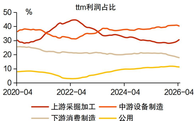
图表 6：4 月上游利润占比提升、中下游承压
