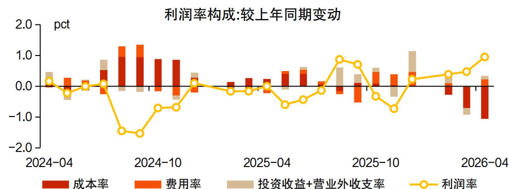
图表 5：4 月利润构成中，降本贡献较大，其次为投资收益改善
