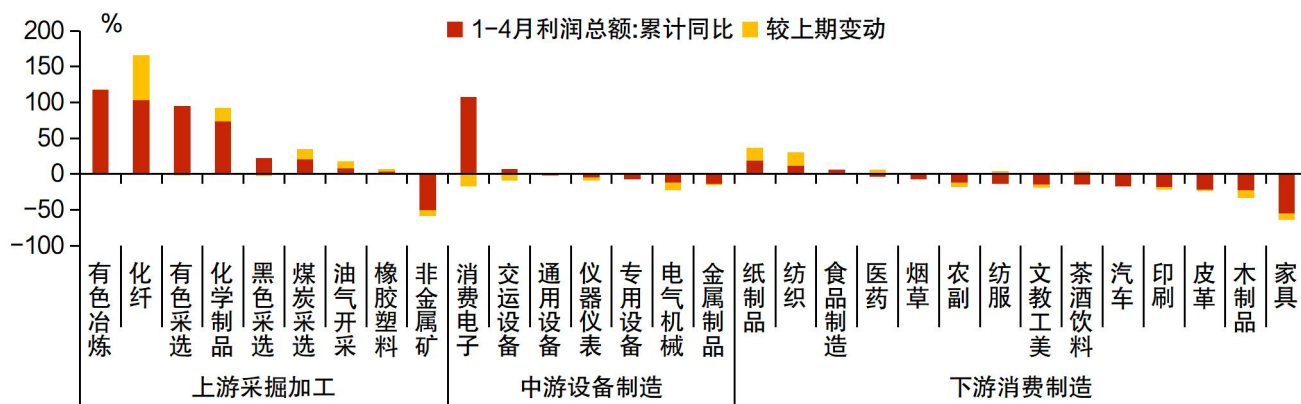
图表 9：4 月化纤、化学制品、煤炭采选、纺织等行业利润边际改善
