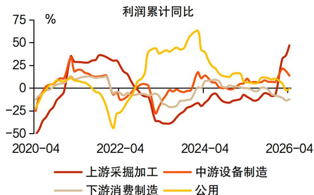
图表 7：4 月上游利润增速向好，中游有所回落
