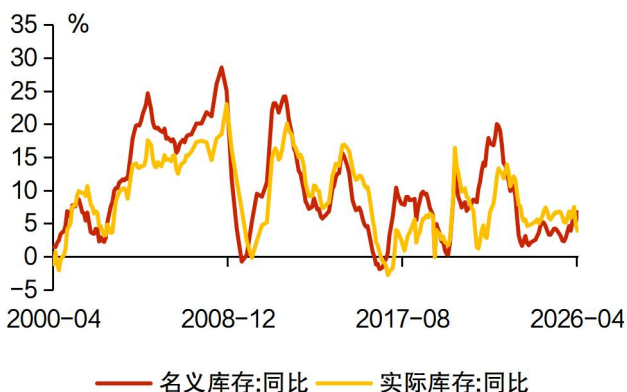
图表 10：4 月名义库存向上、实际库存向下
